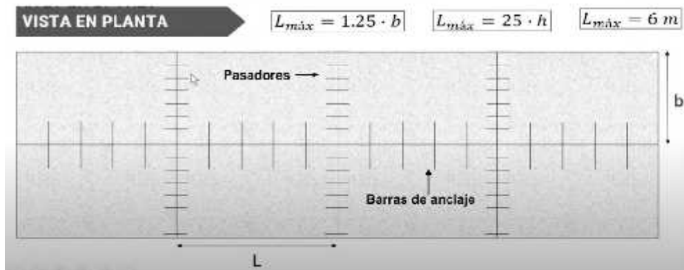
Figura 1. Losa de concreta vista en planta
