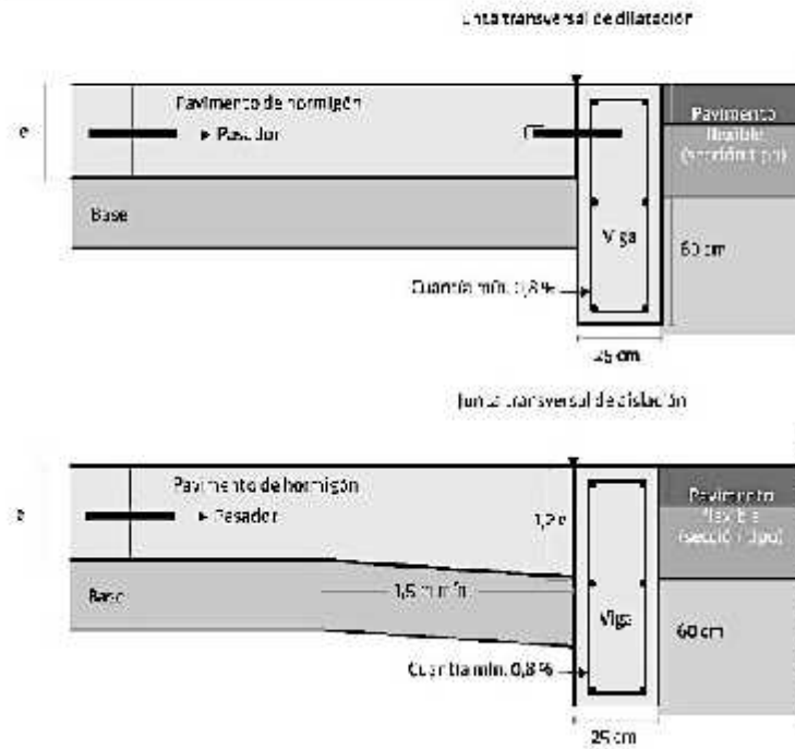
Figura 5. Transición con pavimentos flexibles
